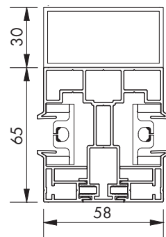
Koppelzijgeleider KU (met uitdiepingsprofiel)
